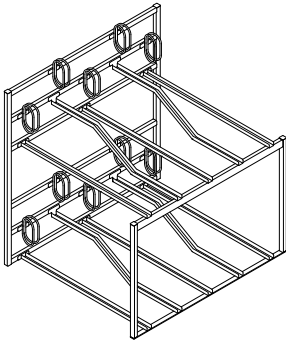
HH20 Etage 10
